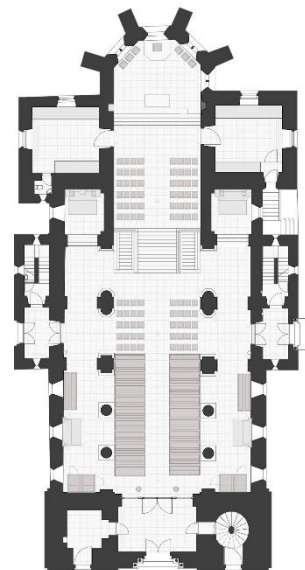
12. kép székesegyház alaprajza
