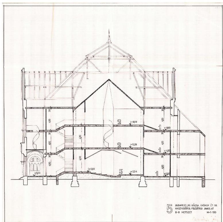
Dózsa György útra merőleges metszet 36
