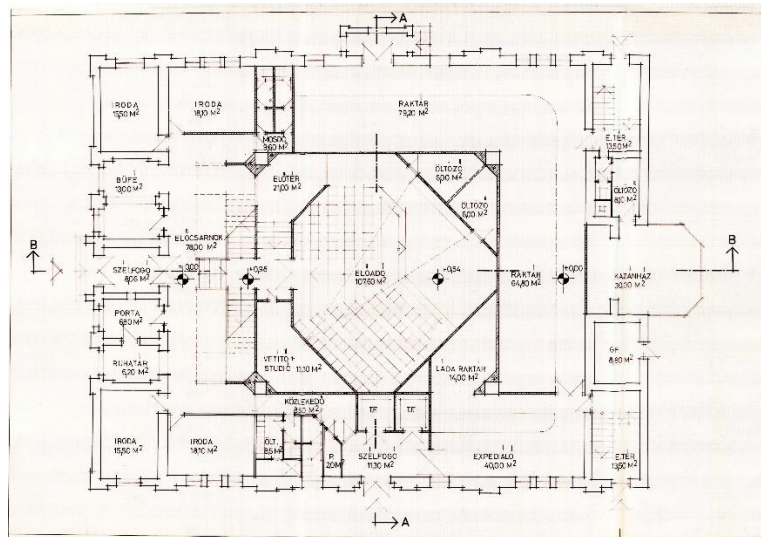
Földszinti alaprajz 33
