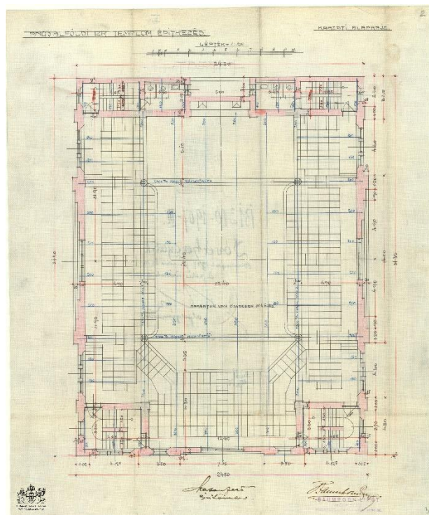
Karzsztint alaprajza 1
