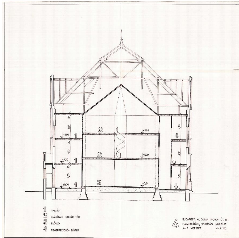
Dózsa György úttal párhuzamos metszet 35
