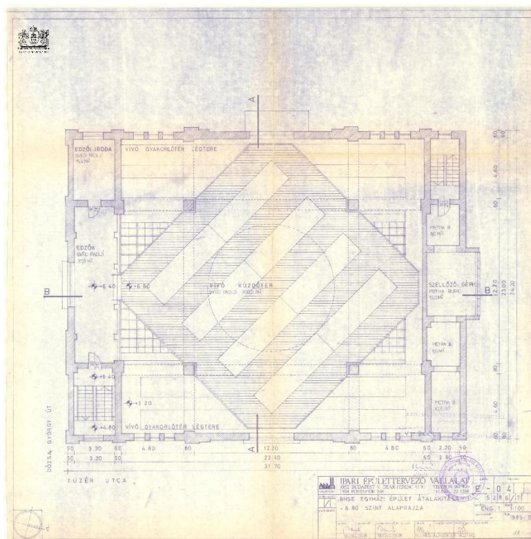
A vívócsarnok második szintjének alaprajza 26
