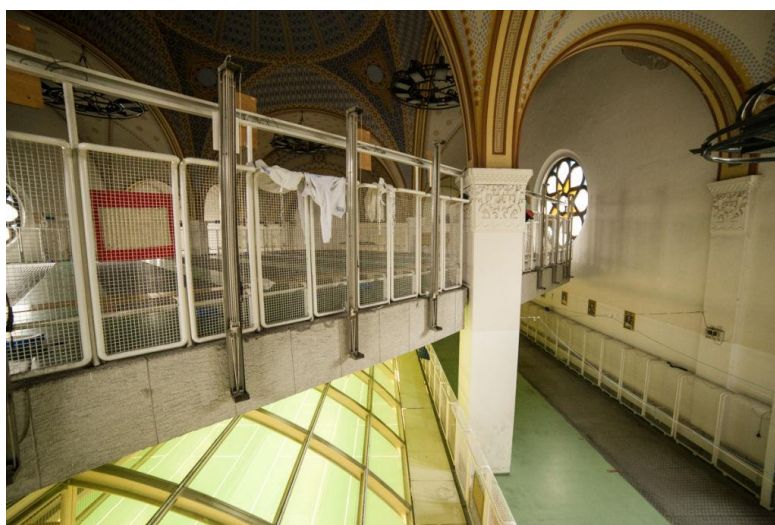
A legfelső szint elforgatott födeme, alatta a karzat szintje, mellette-alatta a földszinti terem 27
