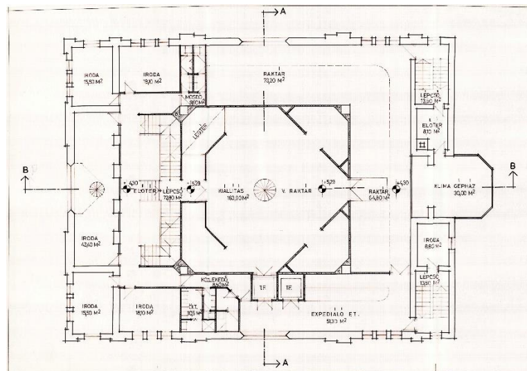
Első szint alaprajza 34
