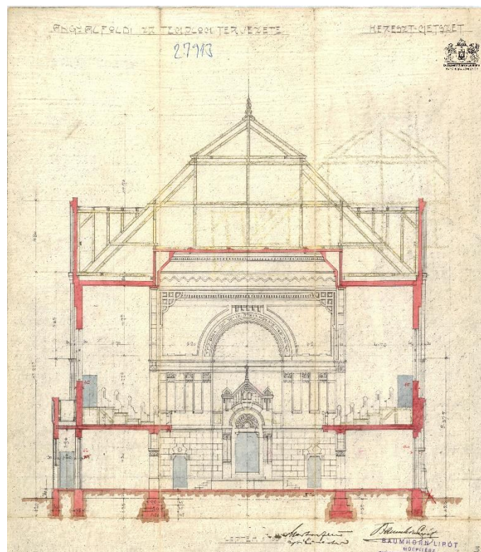
Homlokzati rajzzal párhuzamos metszet 12
