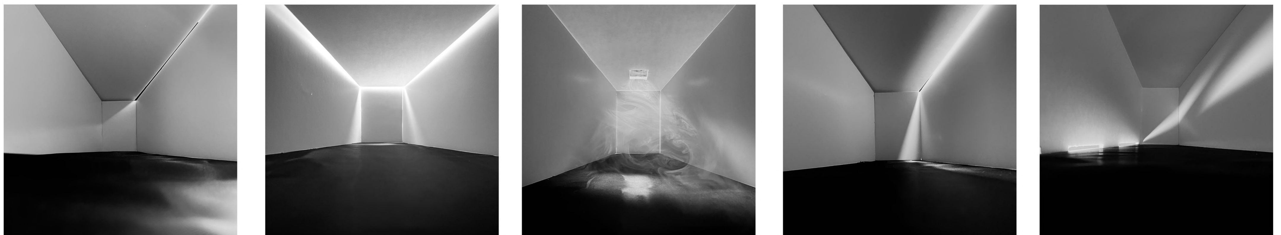
Tér-Fény kísérletek
