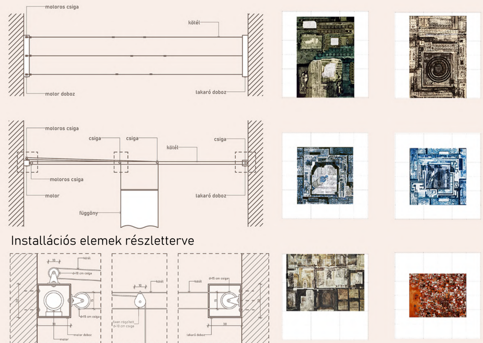
Működési vázlat
