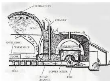
29. ábra: Hypocaustum metszet
