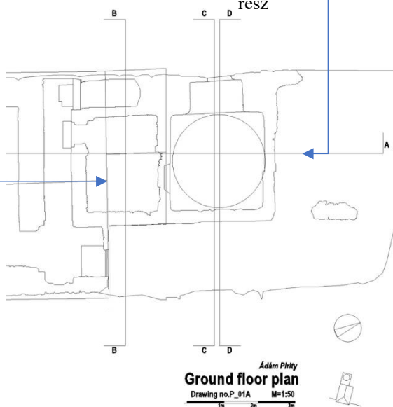
52. ábra: Pontfelhő segítségével feltérképezett alaprajz
