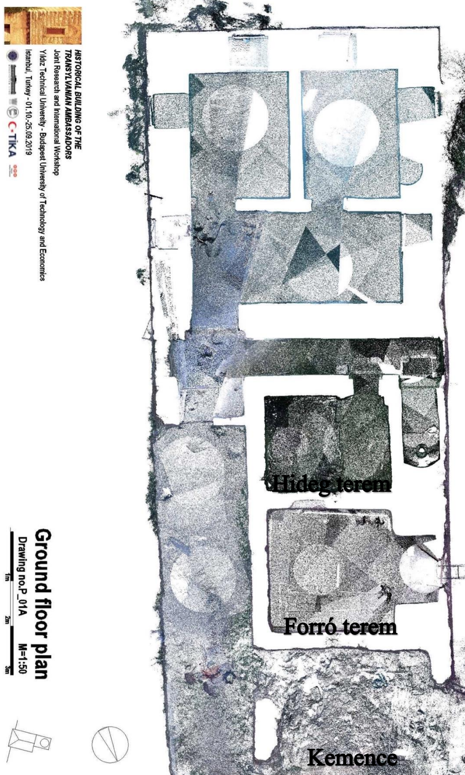
55. ábra: Hamam elrendezése a kutatás alapján
