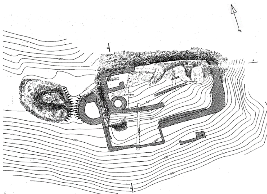
35. Szanda alaprajza
