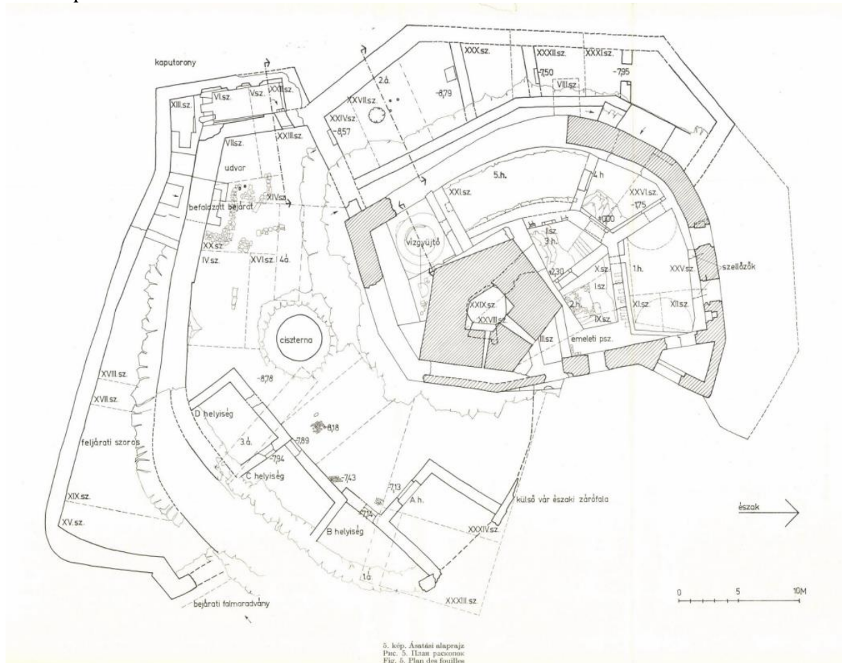
54. Hollókő ásatási alaprajza (Ambrus-Kozák É., 1972. 5. kép)
